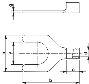
Maßzeichnung
