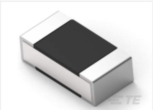
TE Part #6-2176310-0 RP 1E 0.1W 442R 0.1% 25PPM 1K RL
