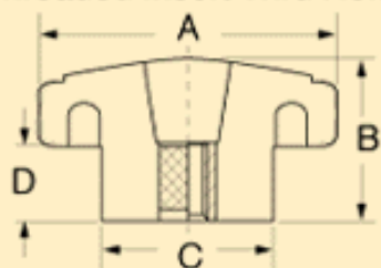
Projecting Stud
