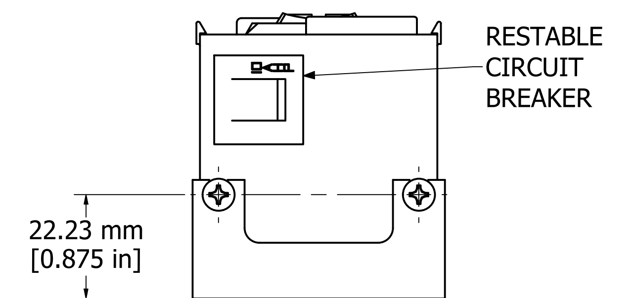
VIEW A-A
