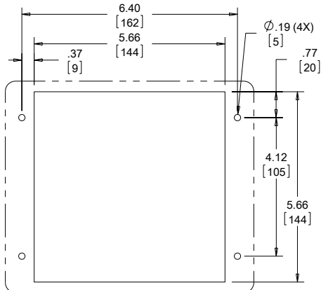
FAN GRILLE OUTLINE
