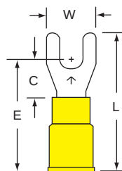
33-8-P Stud Size 8 Wire Range 12-10
