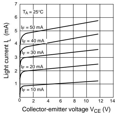
EE-SX1035
