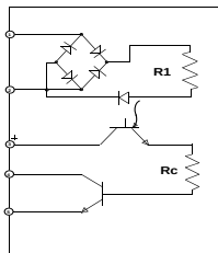
AC/DC INPUT
