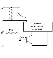
AC OUTPUT
