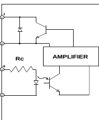
DC OUTPUT
