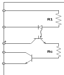
DC INPUT
