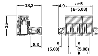
MSTB 2,5 HC/...-STF(-5,08)
