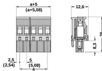
MVSTBW 2,5 HC/...-STF(-5,08)
