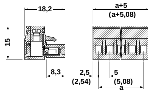
MSTB 2,5 HC/...-ST(-5,08)
