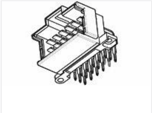
TE Part #9-966140-4 MESSERLEISTE 9P
